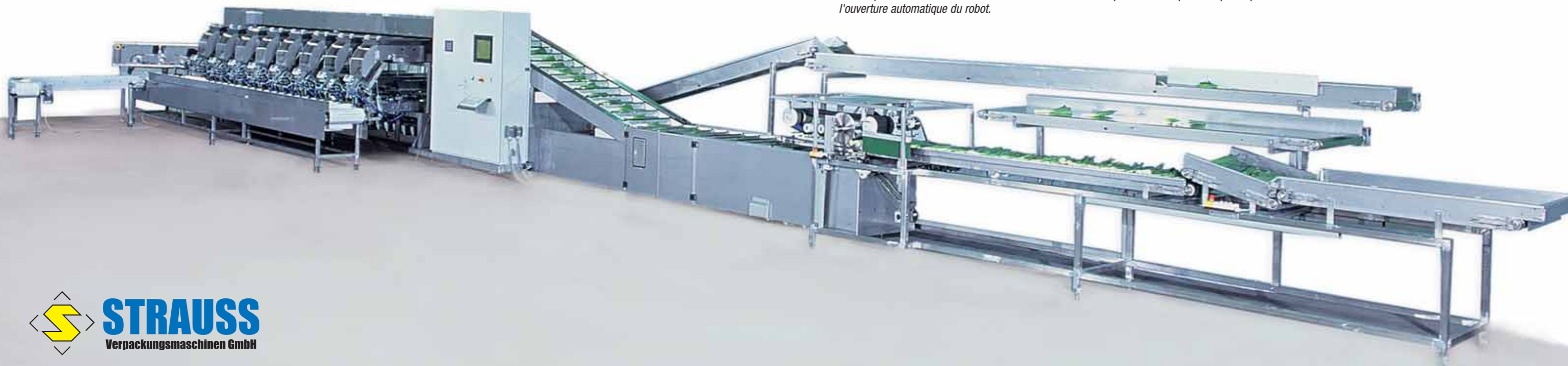
Les unités de poireaux pesées sont transportées des tapis transversales aux robots de remplissage. Les coupelles en carton sont amenées des réservoirs et remplies avec les poireaux pesés par l'ouverture automatique du robot.
